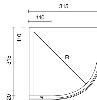
Terminale curvo Curved end unit Накладка закругленная
