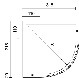
Terminale curvo Curved end unit Накладка закругленная
